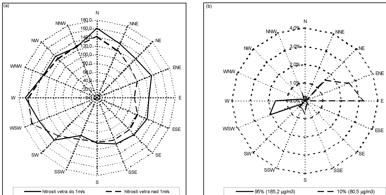
Sl. 5: (a) Roža onesnaženja (povprečne koncentracije ozona) pri različnih hitrostih vetra in (b) vetrovna roža za dve ravni koncentracij ozona (pogostost smeri vetra), Lovran nad Ankaranom.
