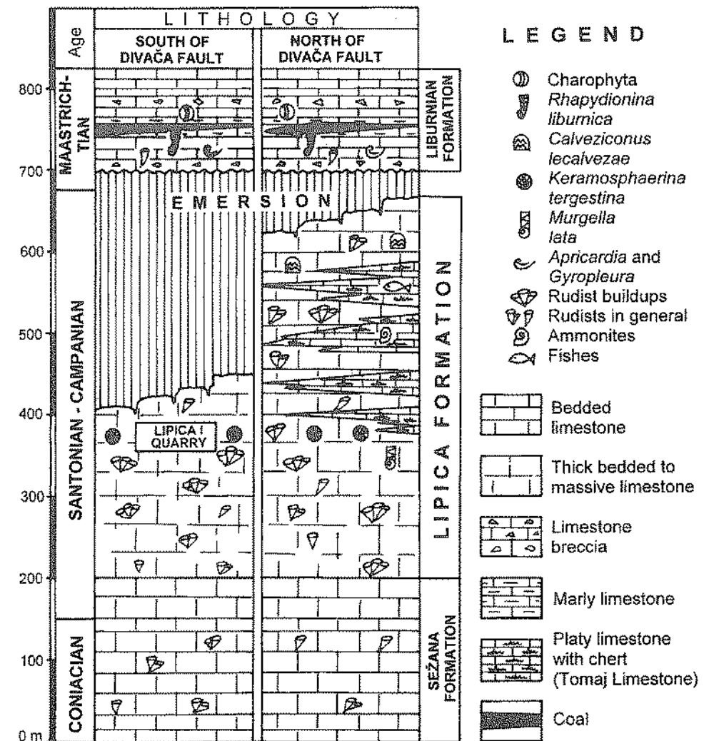
Sl. 3: Primerjava razvoj Lipiške formacije na južnem delu Tržaško-komenske planote. Fig. 3: Comparison of developments of the Lipica Formation in the southern part of the Trieste-Komen plateau.
