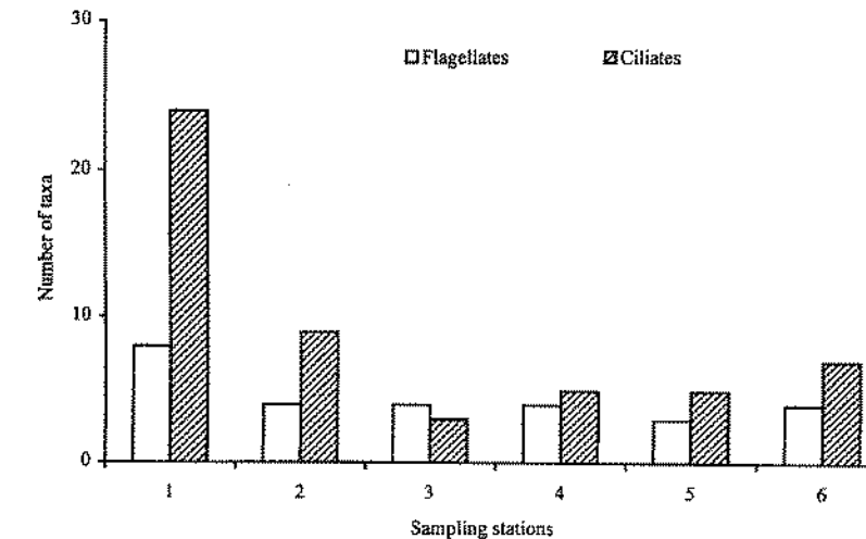
Fig. 2: Number of taxa of Ciliates and Flagellates in six sampling stations of Venice Lagoon in May 1995. Sl. 2: Število taksonov migetalkarjev in bičkarjev na šestih vzorcih postajah v Beneški laguni maja 1995.
