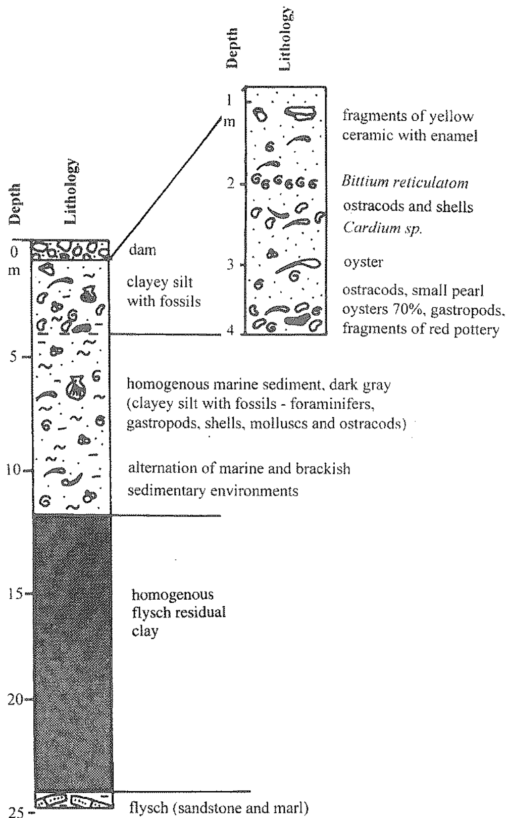
Fig. 4: Borehole Bonifika: lithological succession. Sl. 4: Litologija vrtine Bonifika v Koprju.
