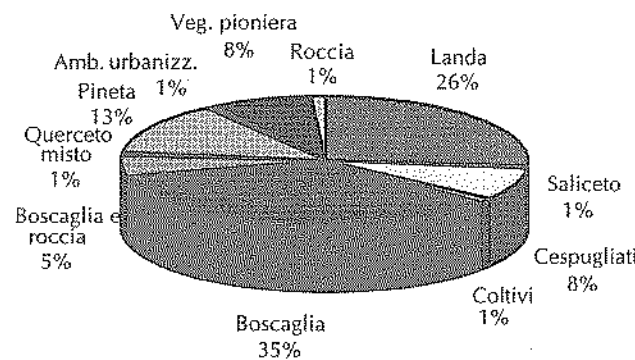
Fig. 2: Ambienti dell'area di studio. Sl. 2: Tipi habitatov na obravnavanem območju.
