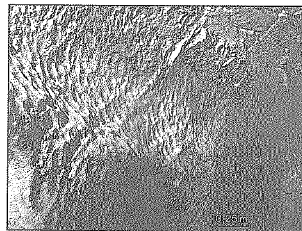
Fig. 4a: Old scallops in Južni Rov. Sl. 4a: Stare fasete v Južnem rovu.
