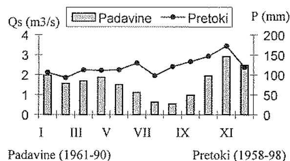
Sl. 6: Povprečni mesečni pretoki Bistrice v obdobju 1958-98 na vodomerni postaji Ilirska Bistrica in povprečne mesečne padavine v obdobju 1961-90 na padavinski postaji Ilirska Bistrica (HMZ RS, 1999; Zupančič, 1995).
