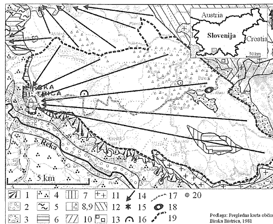
Sl. 7: Geološka zgradba hidrografskega zaledja izvirov in njihovi potencialni onesnaževalci (prirejeno po: Šikić et al., 1972; Petauer et al., 2002; Kovačič, 2001b) Legenda: 1. Pobočni grušč (holocen), 2. Aluvialni nanosi (holocen), 3. Glaciofluvialni sedimenti (pleistocen), 4. Flišni sedimenti: menjavanje glinovcev, laporovcev, peščenjaka, kalkarenitov, breč in konglomeratov (eocen), 5. Svetlosivi in sivi ter sivorjavi do črni apnenci do lapornati apnenci (paleogene), 6. Svetlosivi in beli prekrizalizirani apnenci (zg. kreda), 7. Menjavanje plasti svetlih apnencev in dolomitov (zg. kreda), 8. Svetli apnenci (sp. in zg. kreda), 9. Dolomitno apnena breča (sp. in zg. kreda), 10. Apnenec in dolomit (sp. kreda), 11. Svetlosiv apnenec (zg. jura), 12. Svetlosiv in temnosiv apnenec (zg. jura), 13. Temnosivi debeložrnati dolomit v menjavanju z apnencem (zg. jura), 14. Domnevni podzemeljski dotok vode, 15. Trap-športno strelišče, 16. Kamnolom, 17. Lokalna cesta, 18. Turistično naselje Sviščaki, 19. Predlagana meja vodovarstvenega območja, 20. Kraški izvir.
