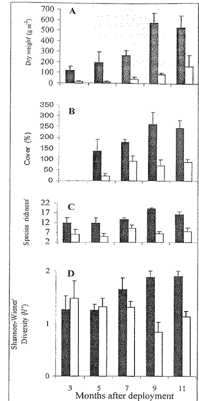
Fig. 1: Characteristics (mean \pm SD) of epi-biota community on artificial substrata near the fish farm (FF - black columns) and reference site (R - white columns), 3 to 11 months after deployment. (A) Dry weight; (B) Cover percentage; (C) Species richness; (D) Shannon-Wiener Diversity ( H' ). Sl. 1: Značilnosti (srednja vrednost \pm SD) epibiotske združbe na umetnih substratih v bližini morske ribogojnice (FF - črni stolpci) in referenčnih lokalitetah (R - beli stolpci), 3 do 11 mesecev po njihovi postavitvi. (A) Suha teža; (B) Pokrovnost; (C) Vrsta pestrost; (D) Shannon-Wienerjev diverzitetni indeks ( H' ).
