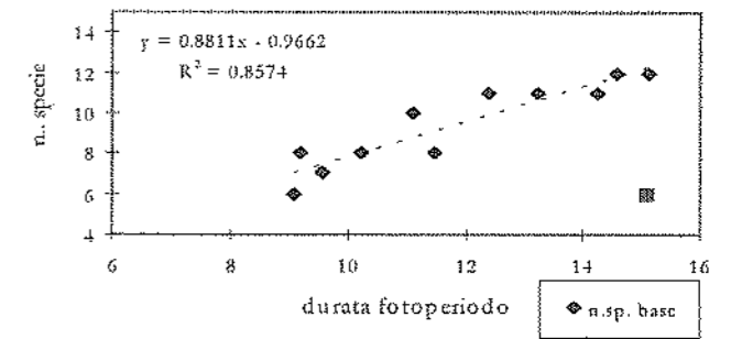
Fig. 5: L'andamento annuale del numero di specie e di durata del fotoperiodo sembra legato da una relazione lineare: y = 0,8811x - 0,9662 .
