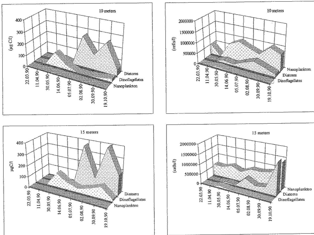
Sl. 6: Razmerje med partikulatnim fitoplanktonskim ogljikom (PPC - \mu\text{gC/l} ) na levi in relativna gostota fitoplanktonskih celic na desni strani na postaji 1 (v globini 10 in 15 m).
