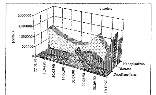
Sl. 5: Razmerje med partikulatnim fitoplanktonskim ogljikom (PPC - µgC/l) na levi in relativna gostota fitoplanktonskih celic na desni strani na postaji 1 (na površju in v globini 5 m).
