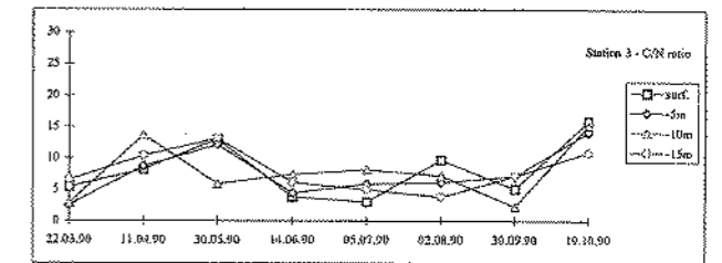
Sl. 4: Razmerje C/N na raziskovalnih postajah.
